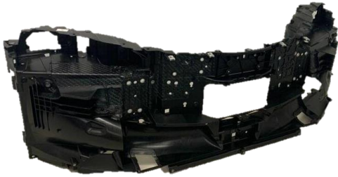
Frontend- modul
